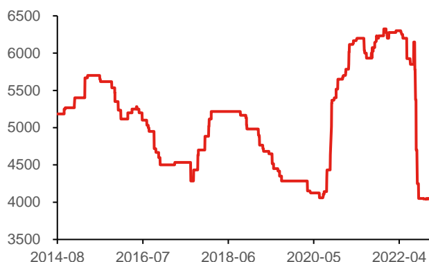
图 15：2018/1/1-2022/12/23 缠绕直接纱均价（元/吨）
