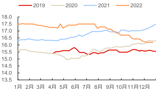
图 9：2019/10-2022/12 玻璃在产产能（万 t/d）
