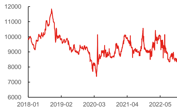
图 36: 2018/1/4-2022/12/23 全国 PP 均价 (元/吨)
