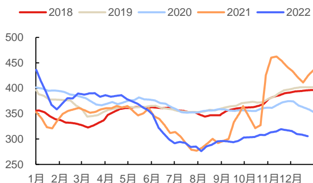
图 27：2018/1/3-2022/12/23 水泥-煤炭价差（元/吨）
