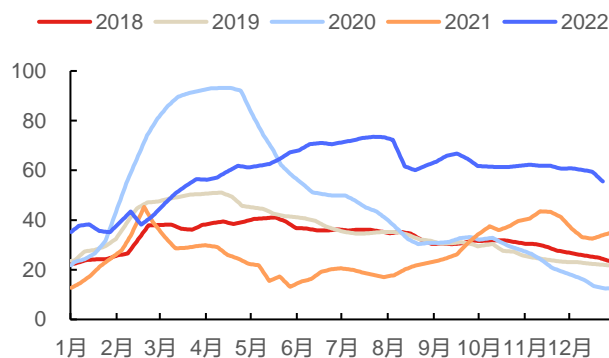
图 10：2018/1/7-2022/12/23 玻璃库存（百万重量箱）
