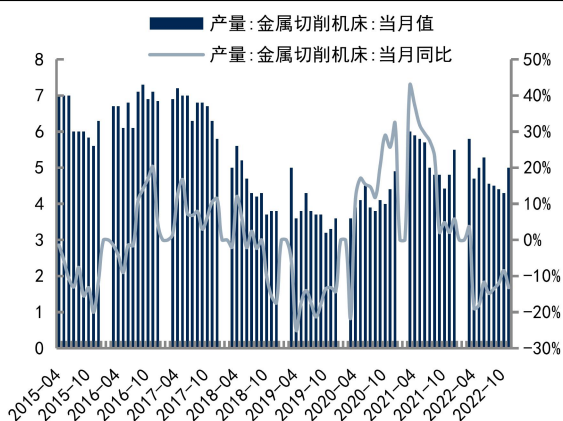
图 17：2022 年 11 月金属切削机床产量同比-13.20%
