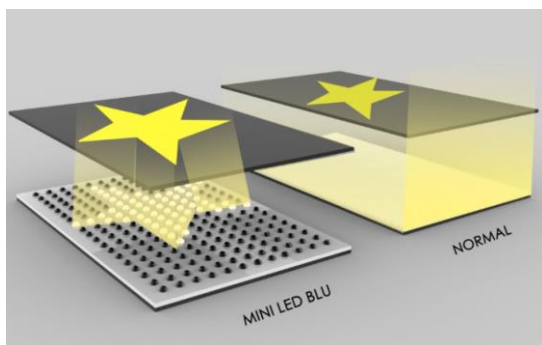
图23：直下式 Mini LED 背光独立控光区域多，提升画面对比度、抑制光晕的状况，面板亮度高、色域广
