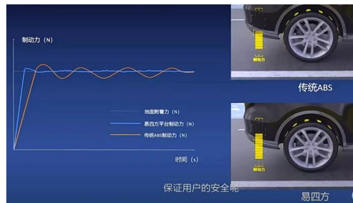
图表 9 易四方与传统 ABS 驱动对比
