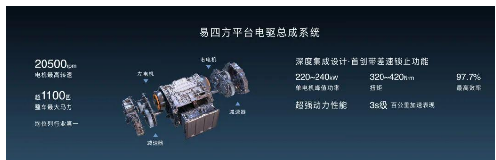
图表 7 易四方平台电驱总成系统
