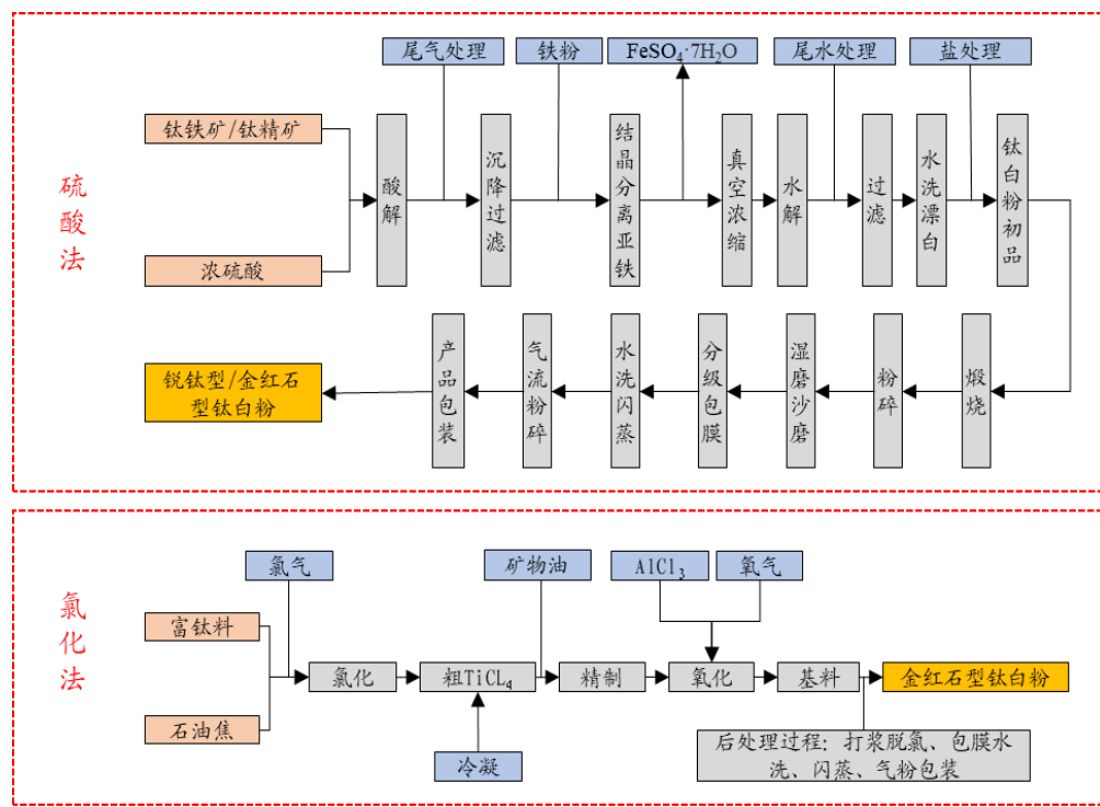
图11：硫酸法与氯化法为钛白粉生产的主流工艺
