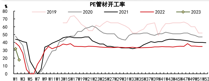
本周PE管材开工率显著回落
