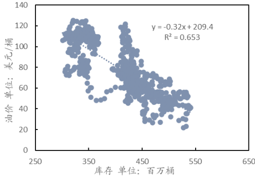
图 25: 2010-2023.1 美国商业原油库存与油价相关性
