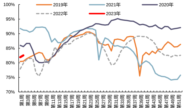
图 26：全国 247 座高炉产能利用率（%）
