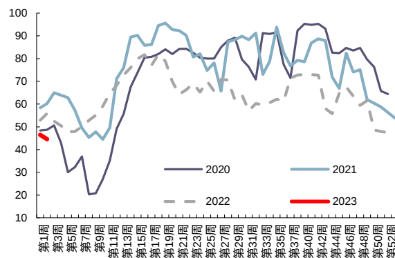
图 30：全国水泥周开工率（%）
