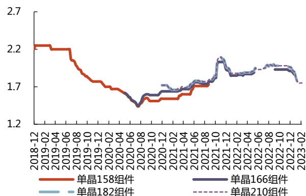
图 35：截至 2023/2/8，光伏组件价格略有下降（元/W）
