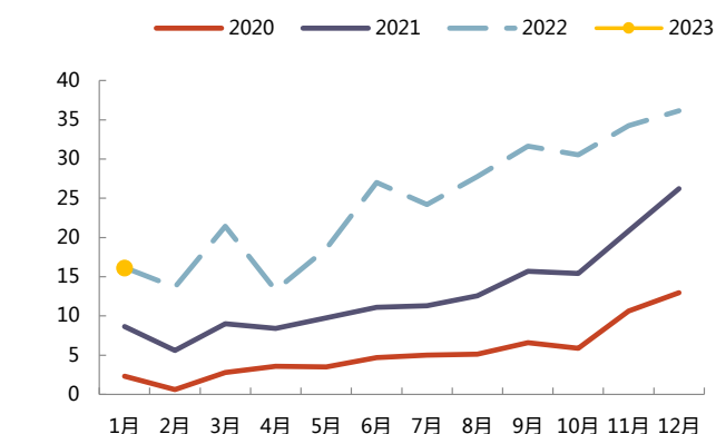
图 30：2023 年 1 月份动力电池装车量当月值 16.1GW
