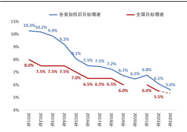
图 3: 2011-23 年各省加权后目标增速与全国目标增速对比
