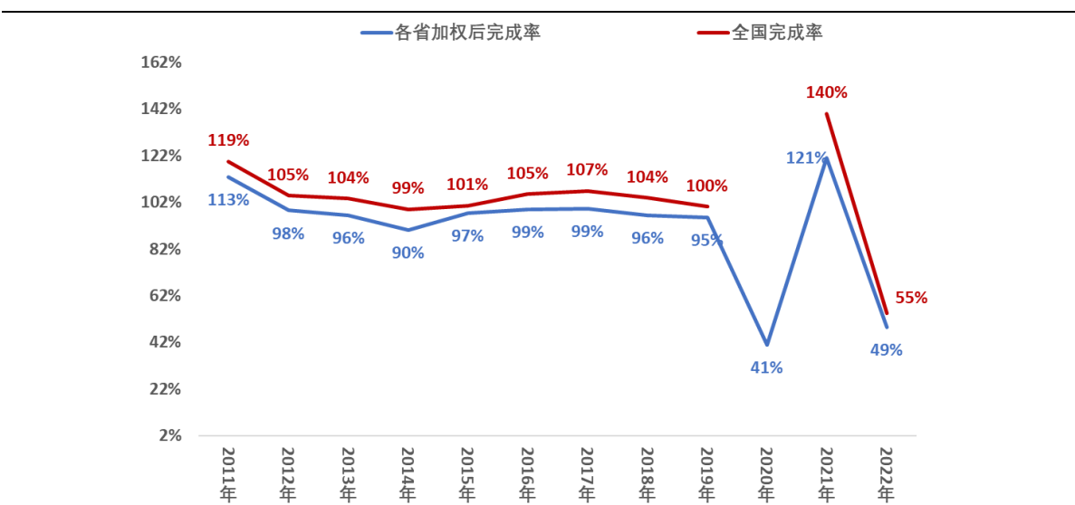
图 5: 2011-22 年各省加权后目标增速完成率与全国目标增速完成率对比
