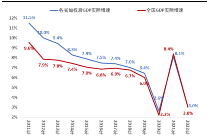
图 4: 2011-22 年各省加权后实际增速与全国实际增速对比
