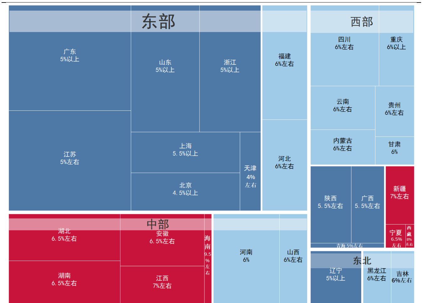
图1：2023年各省区市GDP目标增速分布情况
