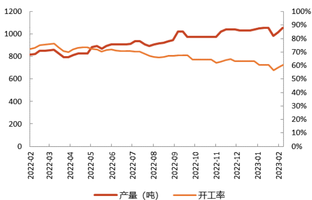
图 19：我国碳纤维产量、开工率（吨）
