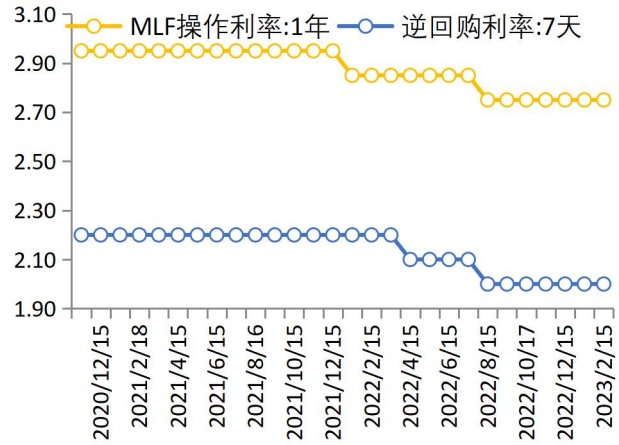
图 2: 政策利率 (%)
