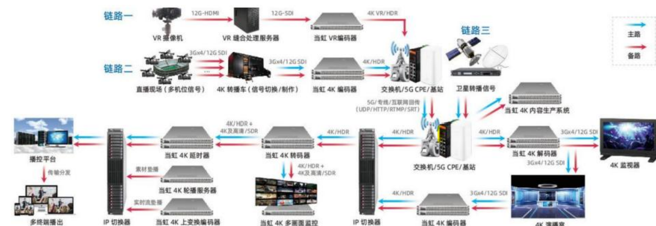
图 25：5G+4K/8K 多场景现场直播解决方案
