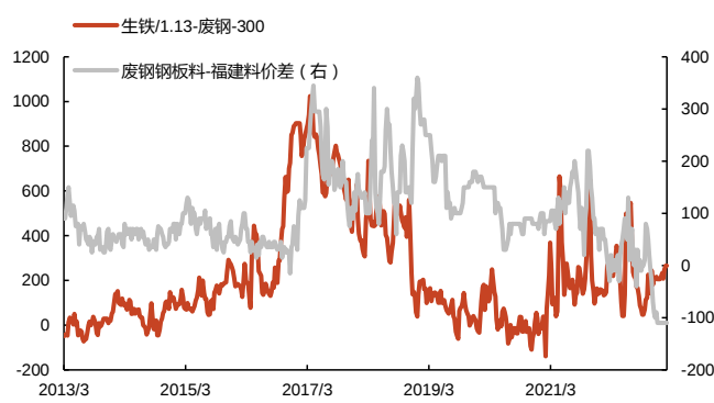
图 86：两种炉料及废钢的价差（元/吨）
