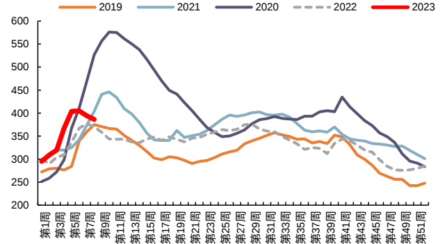
图 22：热轧板卷周度库存（万吨）
