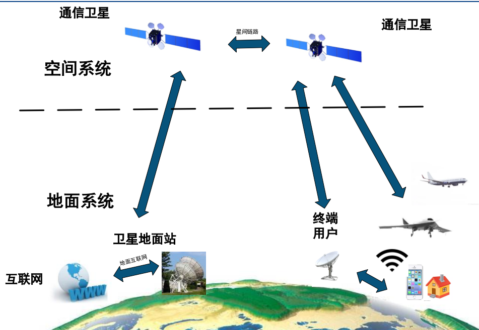
图7 卫星通信（互联网）系统原理示意图
