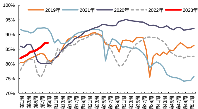
图 26：全国 247 座高炉产能利用率（%）
