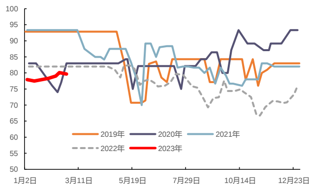
图 45: PVC 开工率 (%)
