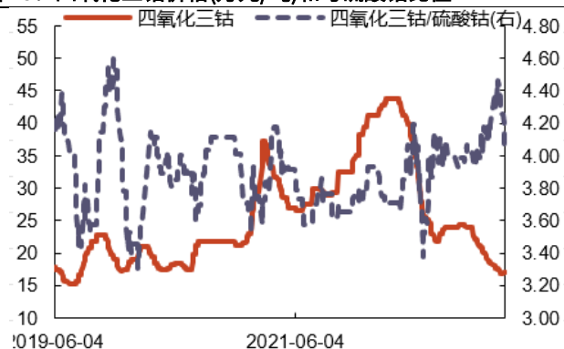
图 73: 四氧化三钴价格(万元/吨)和与硫酸钴比值
