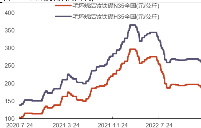
图 51: 钕铁硼价格(元/千克)
