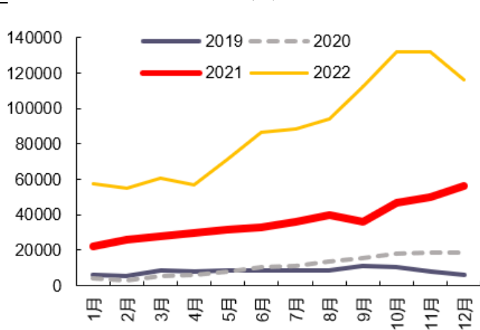
图 34：磷酸铁锂月度表观消费量(吨)
