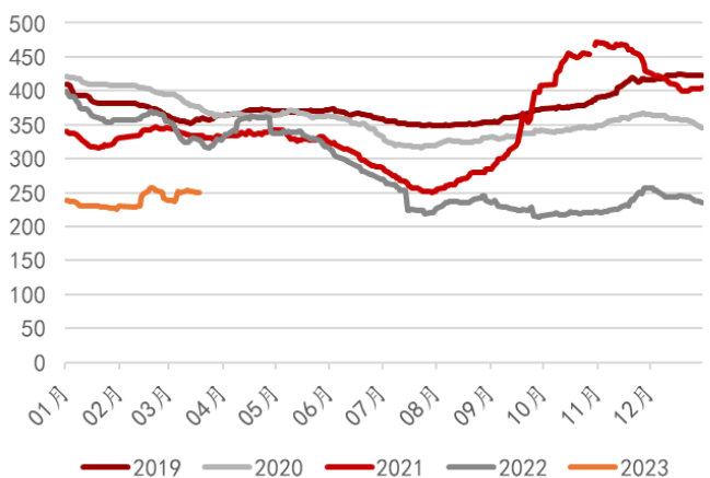
图表23：全国水泥煤炭价格差（元/吨）分年度
