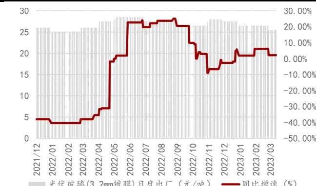
图表45：3.2mm镀膜玻璃价格连续变化（元/平方米）
