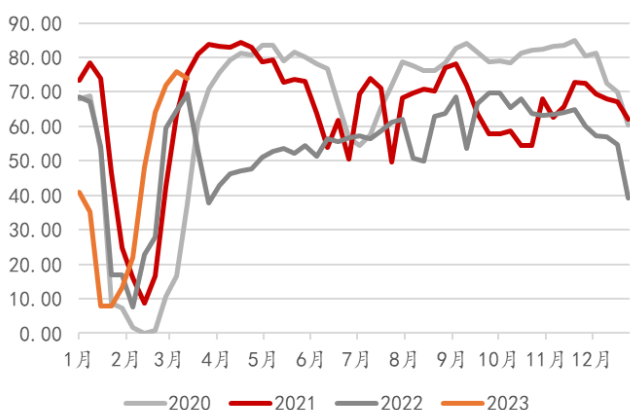
图表37: 华东地区水泥开工负荷 (%)
