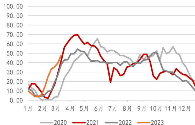
图表36: 华北地区水泥开工负荷 (%)
