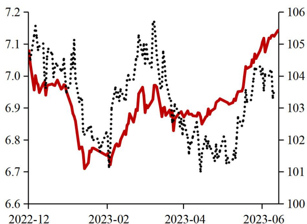
图 27：人民币汇率与美元指数
