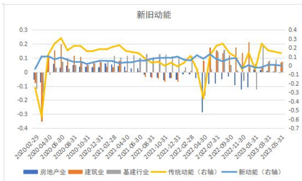
图7. 新旧动能
