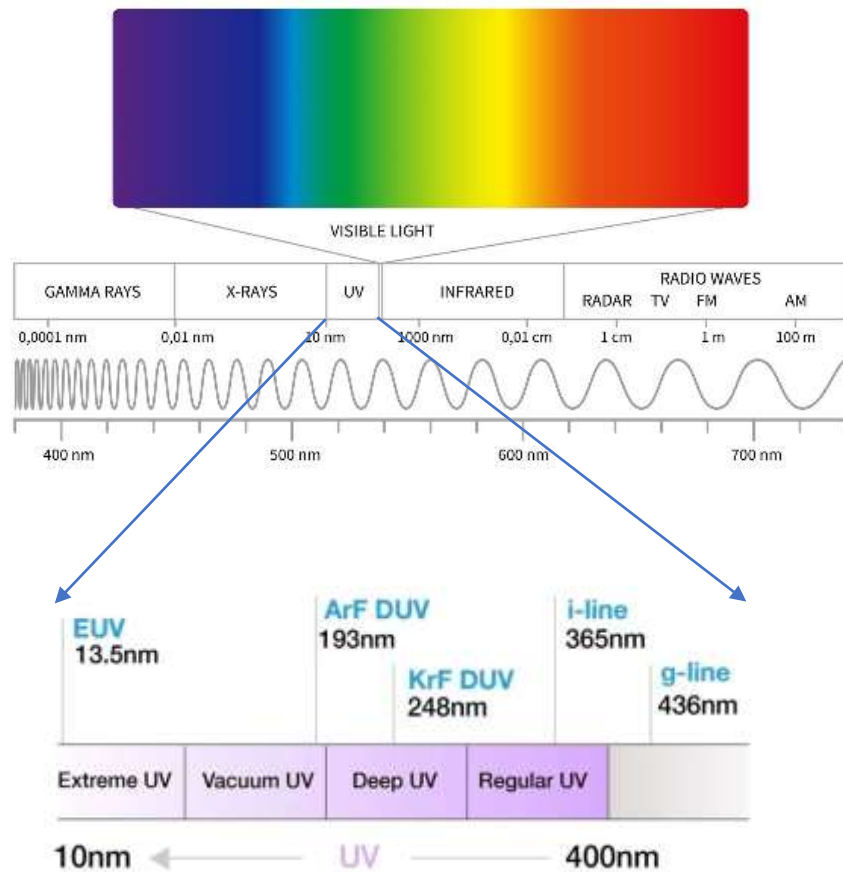
图：光谱图
