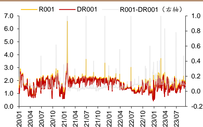
图 6: R001 与 DR001 (%)
