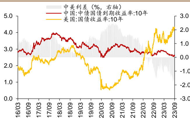
图 8: 中美利差 (%)
