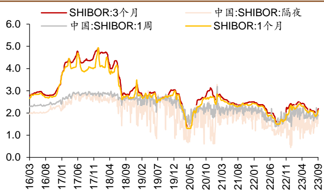
图 5: SHIBOR 利率 (%)
