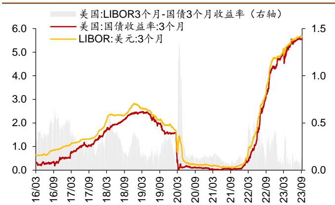
图3:TED利差(%)
