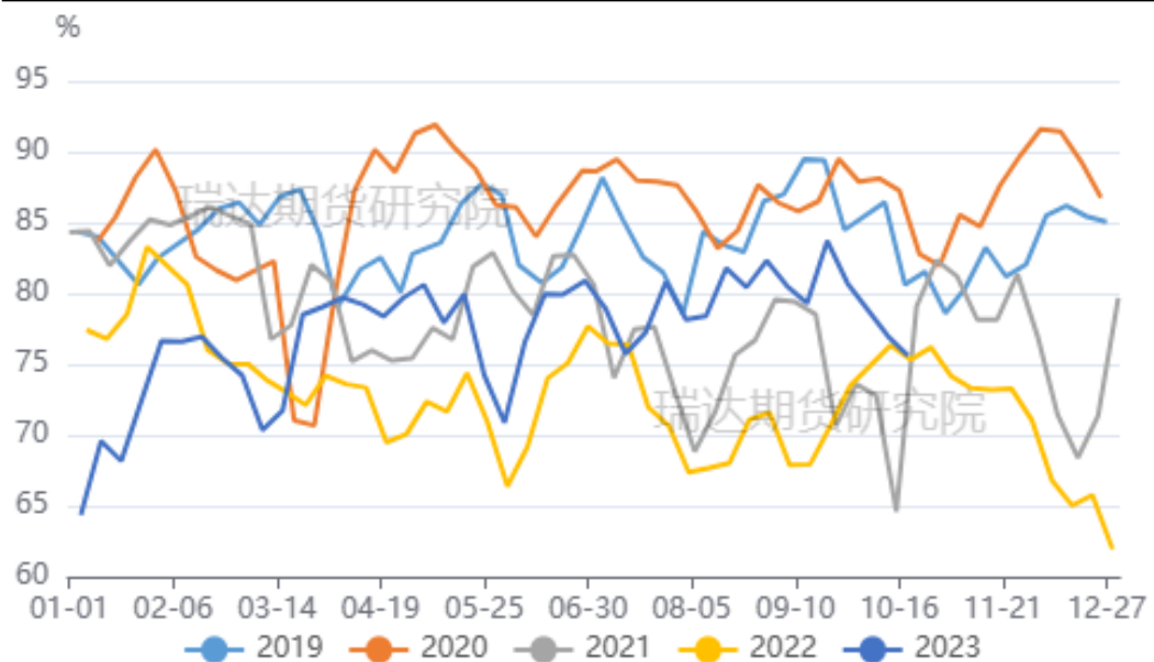
图18、PTA开工率
