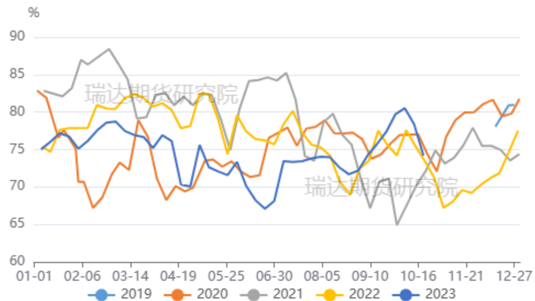
图17、PVC开工率
