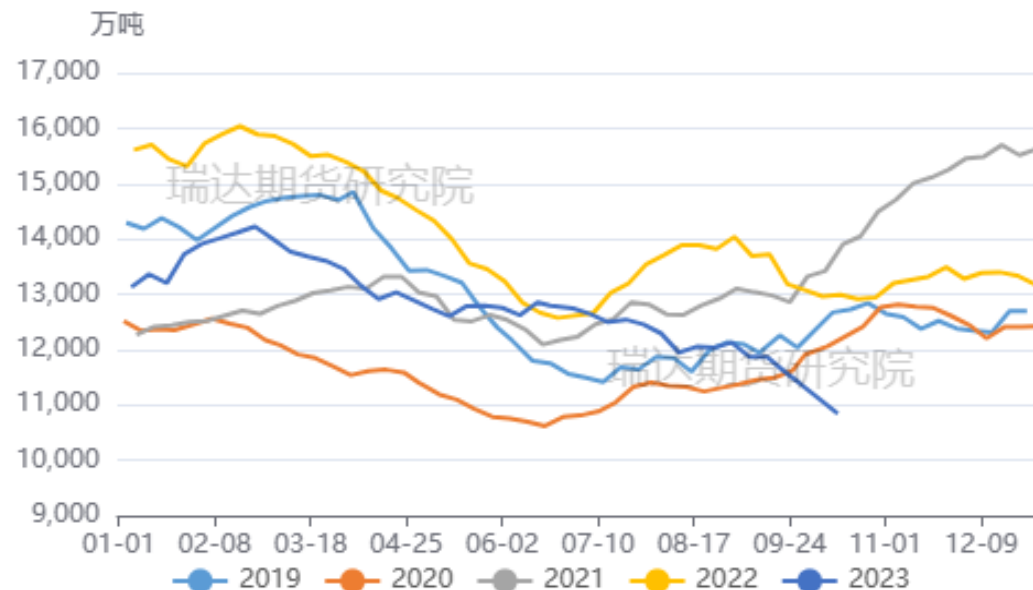
图23、库存：铁矿石
