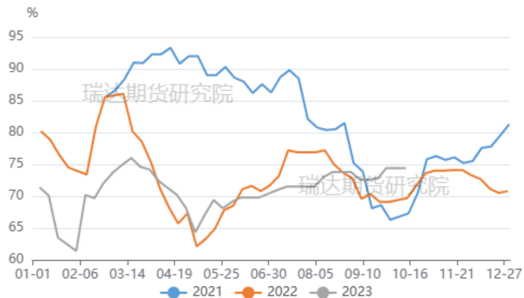
图21、涤纶开工率
