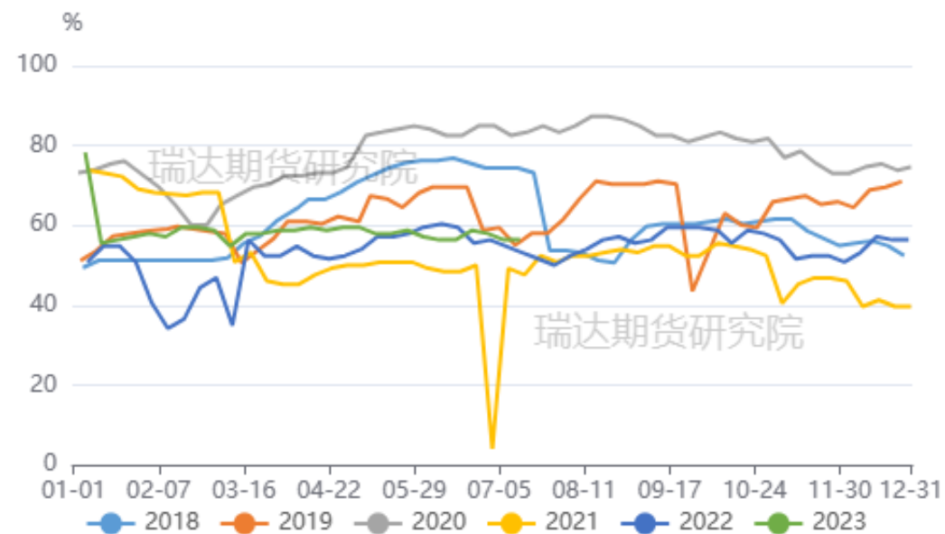
图12、高炉开工率
