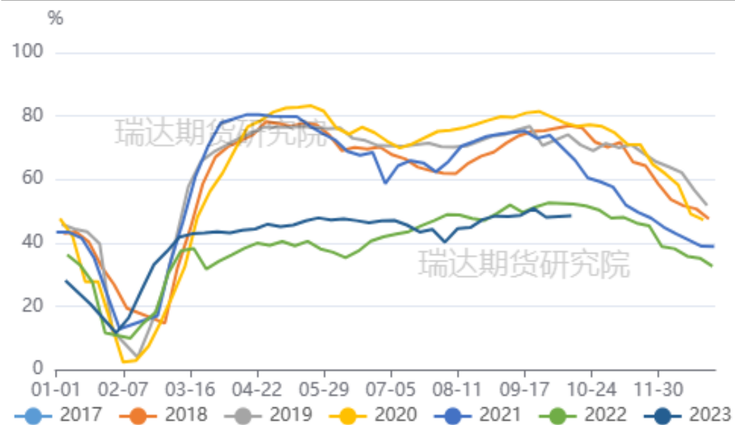
图14、水泥发运率
