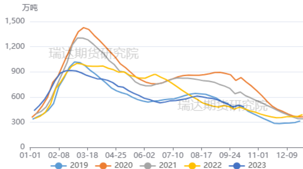
图22、库存：螺纹钢
