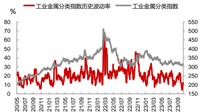
图 30 工业金属波动率指数 8 及标的
