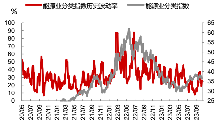
图 28 能源业波动率指数 6 及标的
