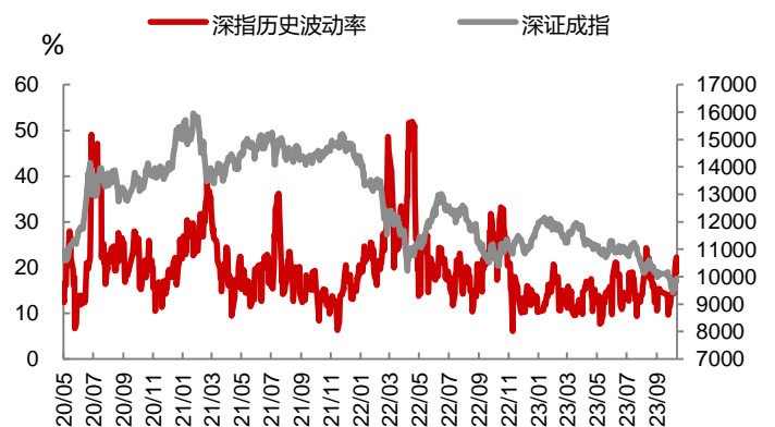
图 14 深指波动率指数及标的走势
