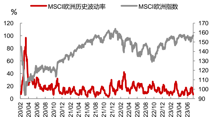
图 36 MSCI 欧洲波动率指数 11 及标的
