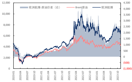
图 25: 原油、欧洲航煤价格及价差 (元/吨, 元/吨)
