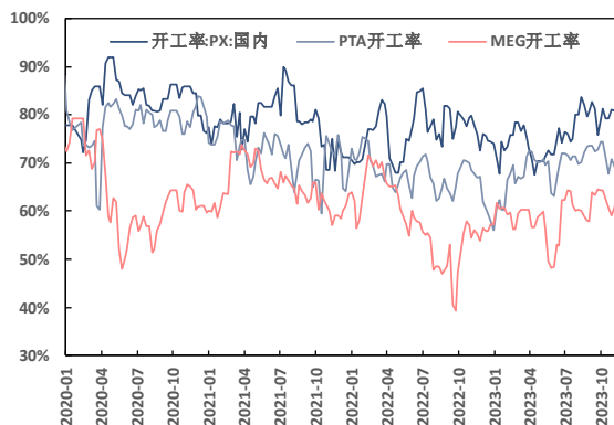
图 41: PX、PTA 和 MEG 开工率 (%)
