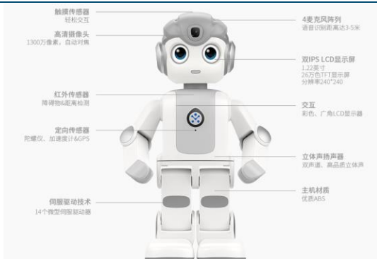
图表57：悟空机器人高 24.5cm，为便携式机器人
