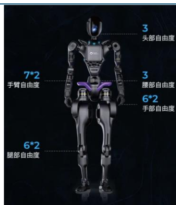
图表69：傅利叶智能 GR-1 全身 44 个自由度
