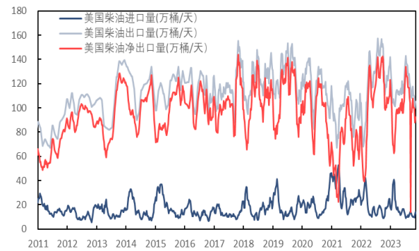
图 56：美国柴油进出口情况（万桶/天）
