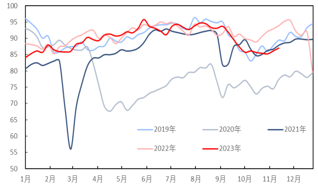
图 23: 美国炼厂开工率 (%)
