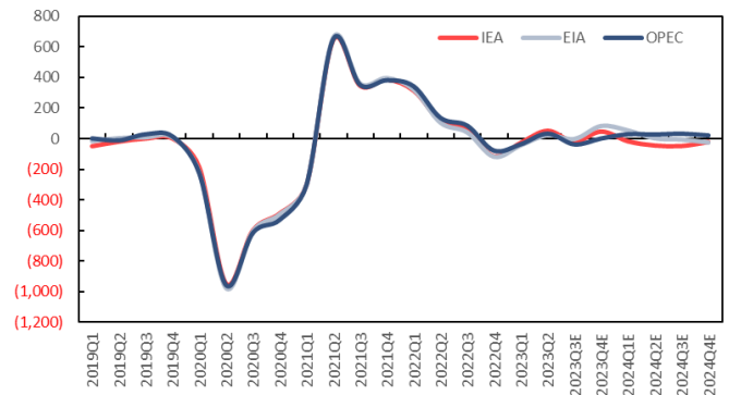
图 72: IEA、EIA、OPEC 对 2019-2024 年 OECD 国家原油需求及预测季度同比增量数据 (万桶/日)
