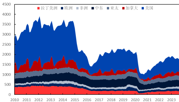
图 21: 2010-2023.10 全球各地区钻机数量 (台)
