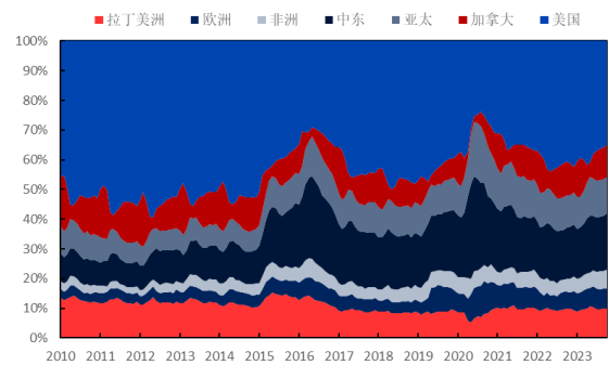
图 22: 2010-2023.10 全球原油钻机数量占比 (%)
