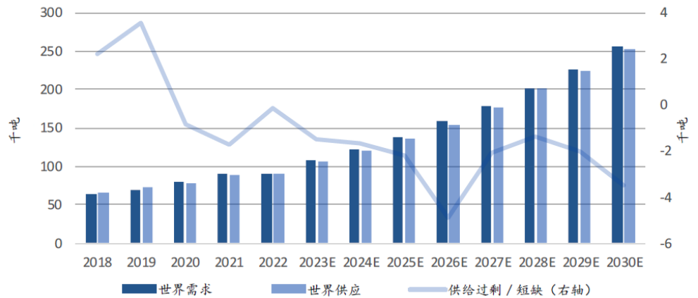
图 36: 全球氧化钨的供需前景趋紧
