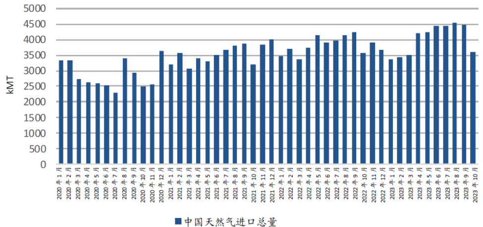
图 39: 中国的天然气管道进口
