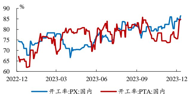
图3：最近两周PX、PTA平均开工率整体上升
