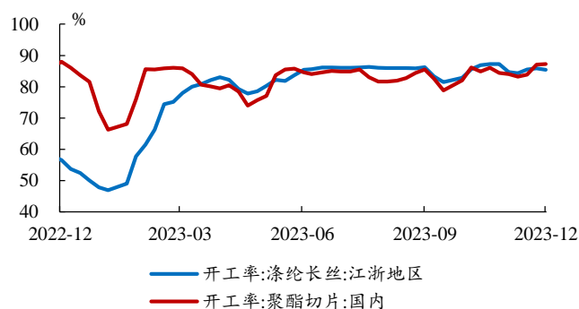
图4：最近两周聚酯切片、涤纶长丝平均开工率整体上升
