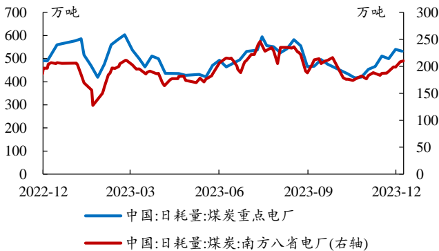
图7：12月前8天电厂煤炭平均日耗较11月回升
