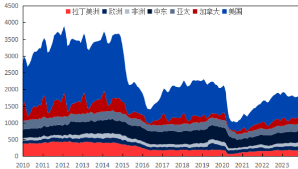
图 21: 2010-2023.11 全球各地区钻机数量 (台)
