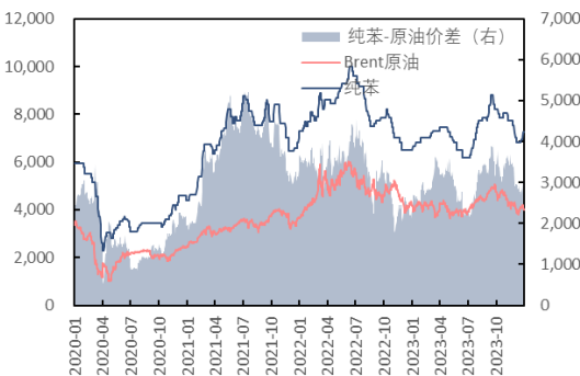
图 31: 原油、纯苯价格及价差 (元/吨, 元/吨)
