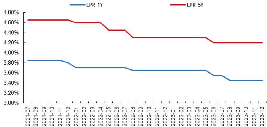
图4: LPR 走势
