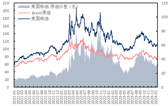
图 44：原油、美国柴油价格及价差（美元/桶，美元/桶）
