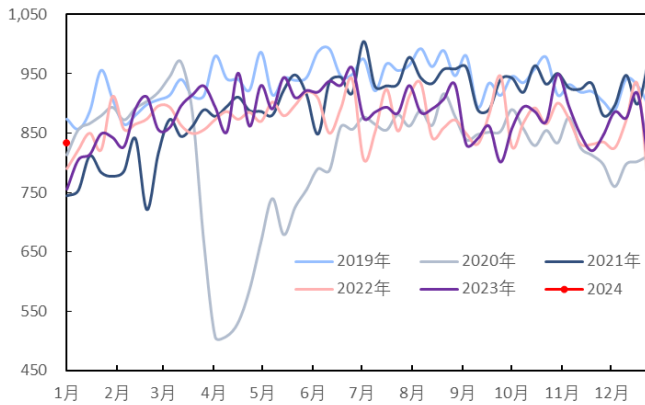
图 56: 美国成品车用汽油消费量 (万桶/天)
