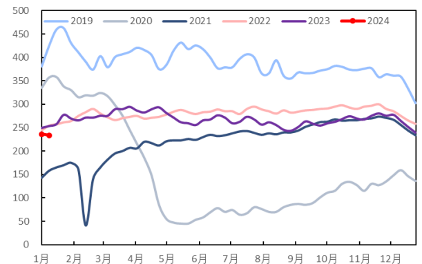
图 21：美国压裂车队数（部）
