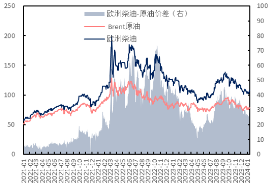
图 47：原油、欧洲柴油价格及价差（美元/桶，美元/桶）
