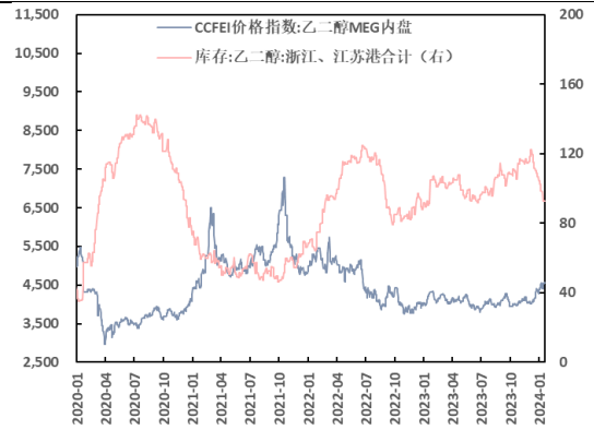
图 42: MEG 价格和华东 MEG 库存 (元/吨, 万吨)
