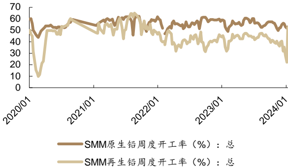
图 25: 2024 年 1 月 19 日，原生铅最新周度开工率为 51.79%，再生铅最新周度开工率为 0.00%
