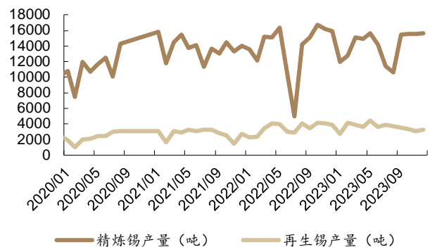
图 36：2023 年 12 月，精炼锡产量 15685 吨，同比减少-1.38%，再生锡产量 3250 吨，同比减少-15.58%
