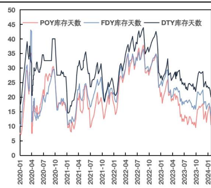
图 50: 聚酯企业的涤纶长丝库存天数 (天)
