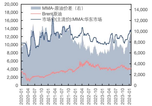
图 38: 原油、MMA 价格及价差 (元/吨, 元/吨)
