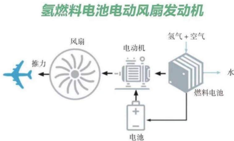
图 7：氢燃料电池电动风扇发动机示意图
