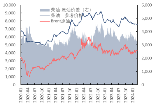
图3：原油、国内柴油价格及价差（元/吨，元/吨）
