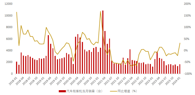
图 13: 汽车起重机销量及增速 (台, %)
