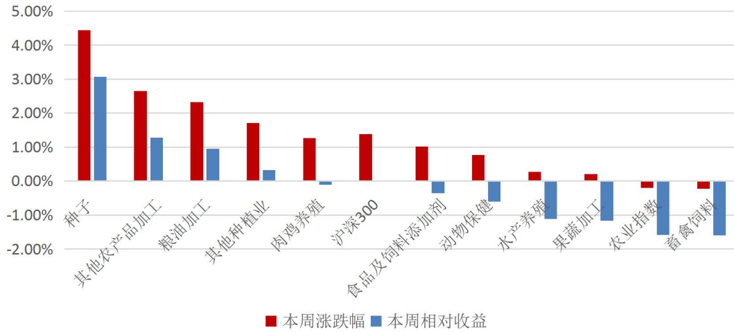
图 5：本周农业各子行业涨跌幅
