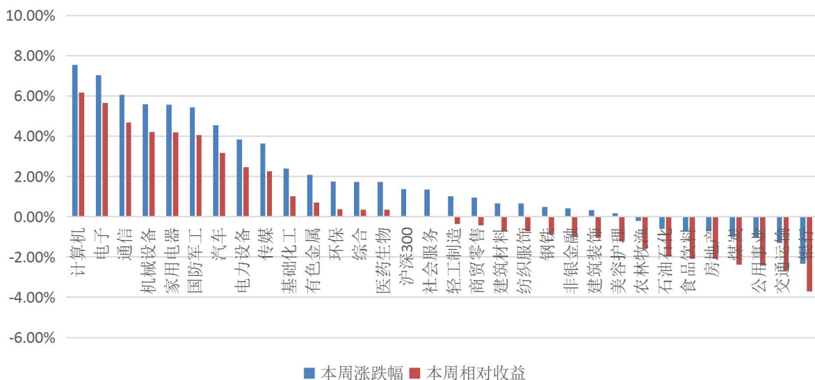
图4：本周各行业板块涨跌幅
