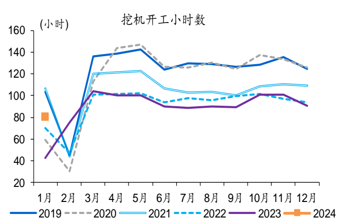
图表26: 2024年1月挖掘机开工小时数约80小时
