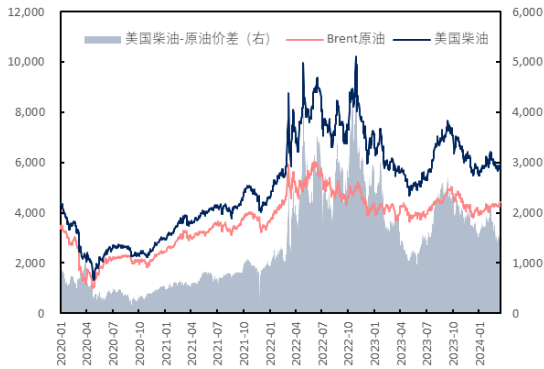
图 15: 原油、美国柴油价格及价差 (元/吨, 元/吨)
