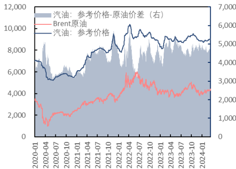
图 5：原油、国内汽油价格及价差（元/吨，元/吨）
