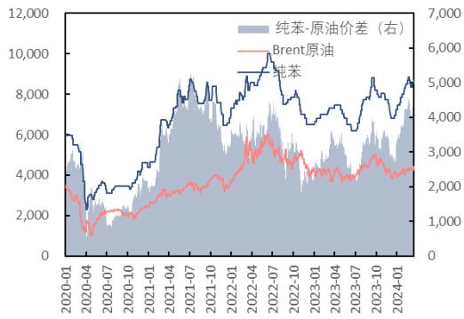
图 31: 原油、纯苯价格及价差 (元/吨, 元/吨)
