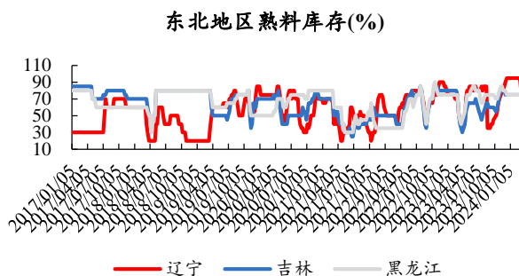
图11：本周辽宁熟料库存持平，吉林、黑龙江均环比下降
