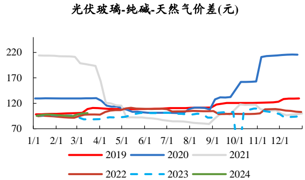
图52: 当前光伏玻璃盈利能力位于2023年同期水平
