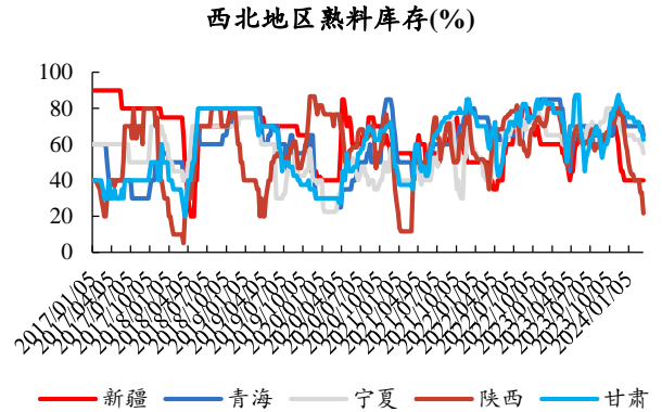
图23: 本周新疆熟料库存环比持平, 其余下降
