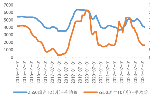
图表 21: 国产及进口 50% 锌精矿加工费
