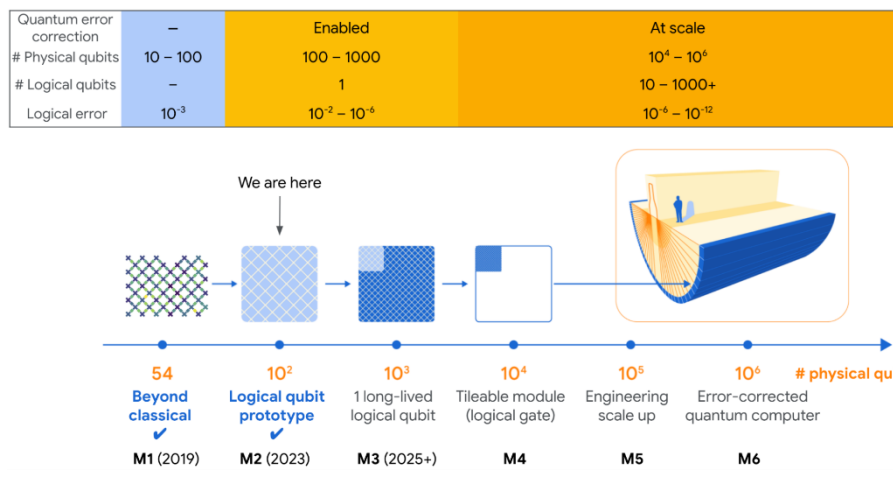
图14：谷歌量子计算路线图
