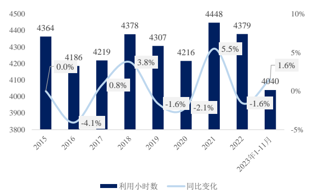
图12: 2015-2023年1-11月火电利用小时
