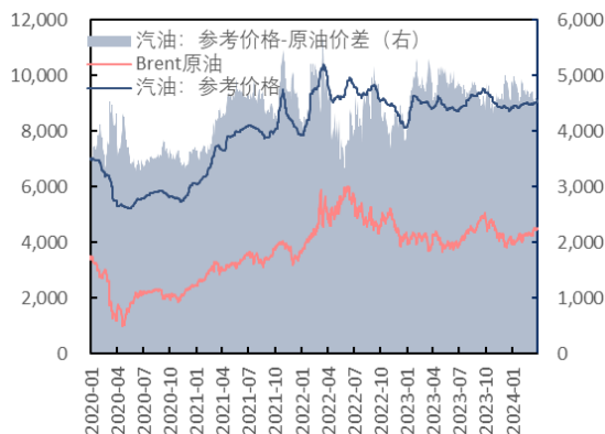
图 5：原油、国内汽油价格及价差（元/吨，元/吨）
