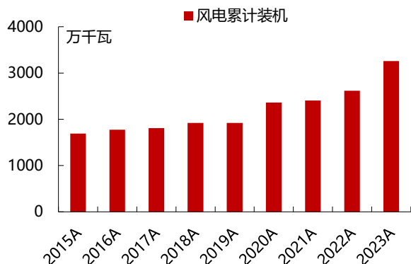
图2：2015-2023 年新疆累计风电装机
